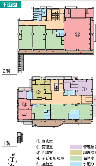
平面図
